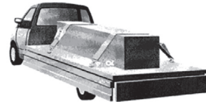
Beispiel Niederzurren
